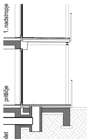
**DELNI PREREZ ZAJEMA ZRAKA PREZRAČEVANJA KLETI
