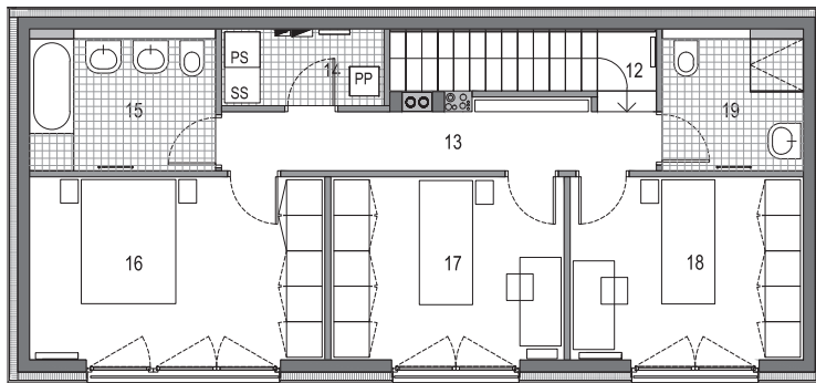
terasna etaža
