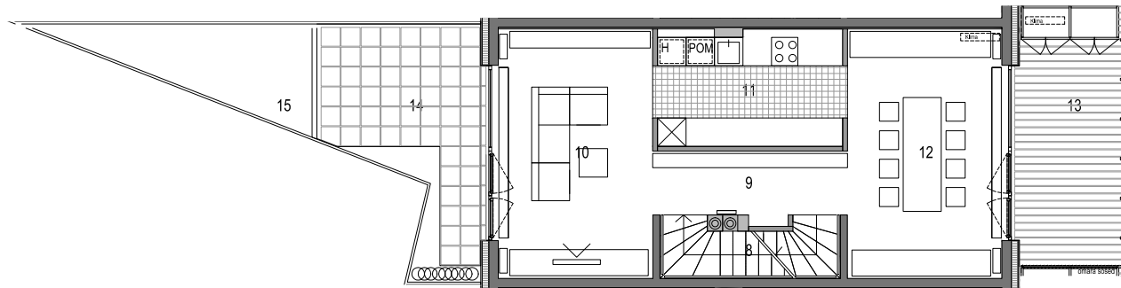
pritličje
