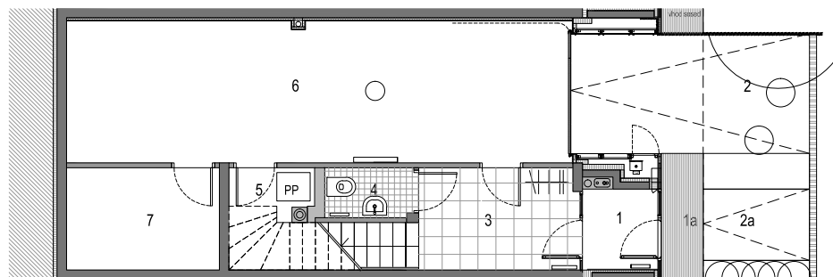
kletna etaža
